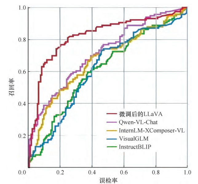
图 5 各模型在测试集上的 ROC 曲线
